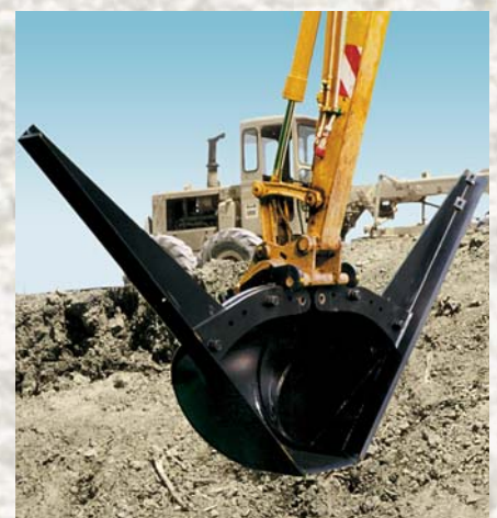
Profielbakken
